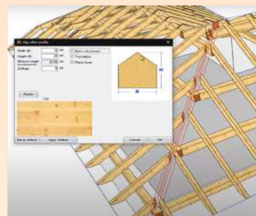
Generazione automatica di travi di displuvio e compluvio personalizzate
